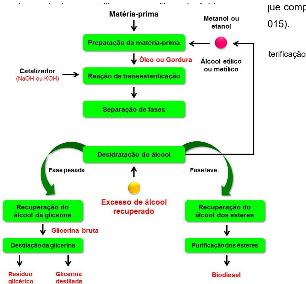
Figura 02: Fluxograma do processo de produção de biodiesel.
