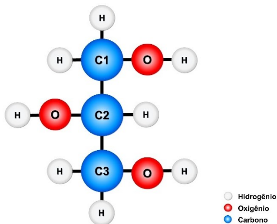
Figura 03. Fórmula estrutural do glicerol (1,2,3-propanotriol)
