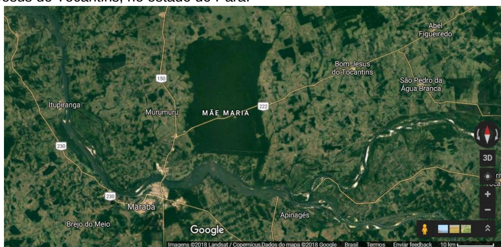
Figura 7 – Imagem via satélite, da Terra Indígena Mãe Maria, localizada no município de Bom Jesus do Tocantins, no estado do Pará.
