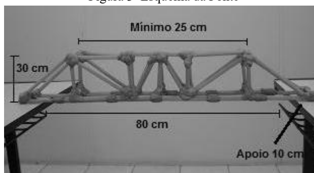
Figura 3–Esquema da Ponte
